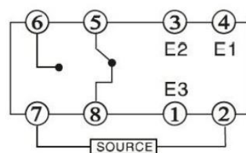
线路图
