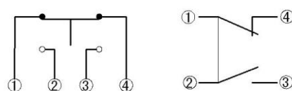
接线方式及回路图
