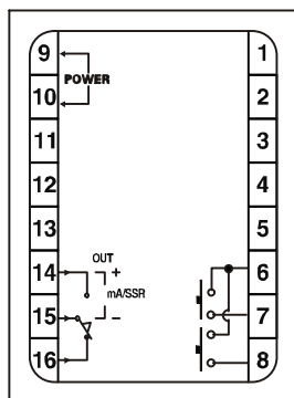
ATR06-B1接线图
