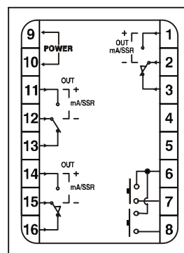
ATR06-B4接线图
