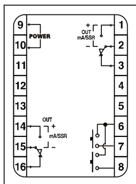
ATR06-B2接线图
