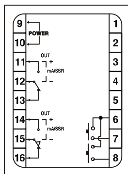
ATR06-B3接线图
