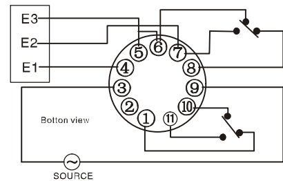
线路图
