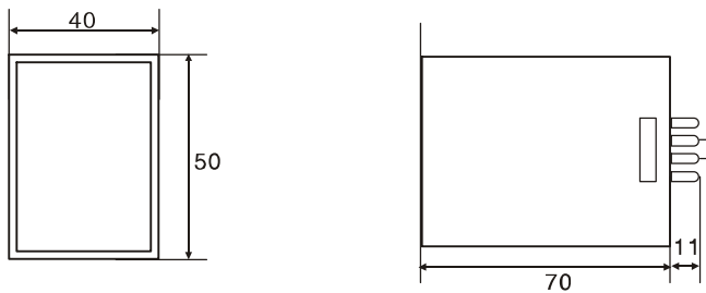
安装尺寸
