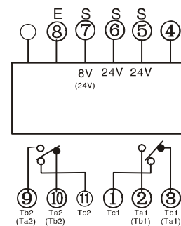
线路图
