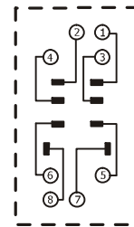
接线图
