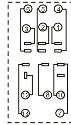
接线图
