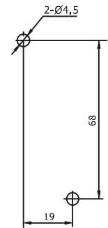
安装孔尺寸
