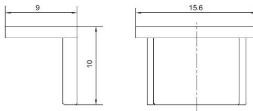
标识卡尺寸
