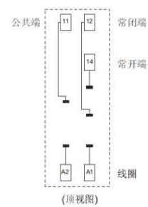
接线图
