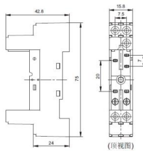
外形图
