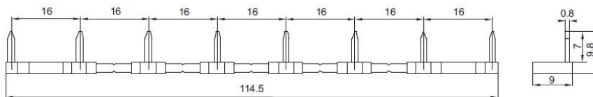
跨接片尺寸
