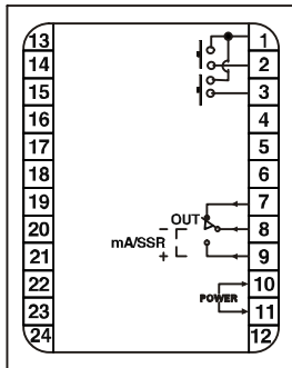
ATR10-B1/ATR11-B1接线图
