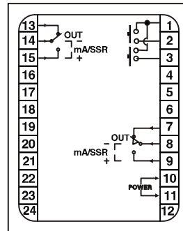
ATR10-A3/ATR11-B3接线图
