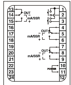
ATR10-B4/ATR11-B4接线图
