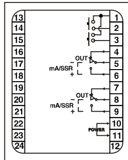
ATR10-B2/ATR11-B2接线图
