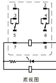
ARN3F-2CL (带发光二极管)
