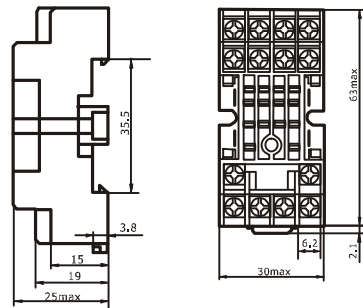
外形图
