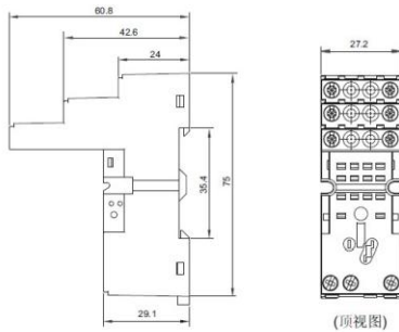
外形图
