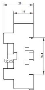
外形图
